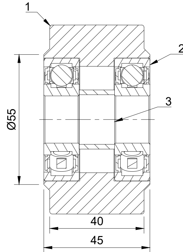
A-A (1:1)
